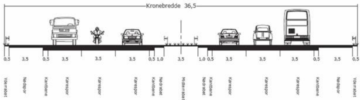
Figur 4.4: Tværprofil 6 sporet motorvej på strækning i åbent land (eks. Stenløse Øst - Måløv)
